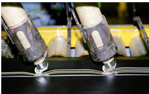
Imagem 1: Marcação das linhas durante a extrusão da banda de rodagem.
