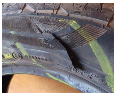
Imagem 1: Exemplo de corte lateral.
